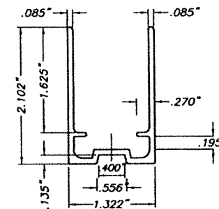
G1 ALTERNATE BAHAMA FRAME SCALE: 1/2" = 1"
