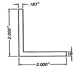
H CORNER KEY 1" LONG SCALE: 1/2" = 1"
